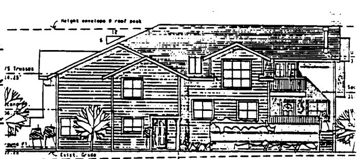
WEST ELEVATION Scale: 1/8"=1'-0"
